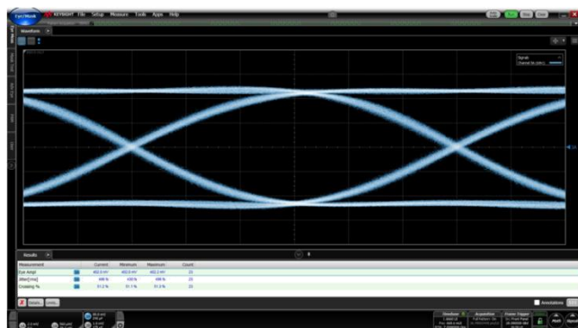
Input Signal @28Gbps
