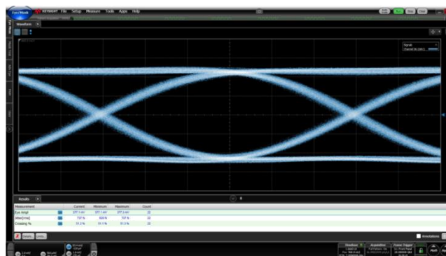
Output Signal @28Gbps
